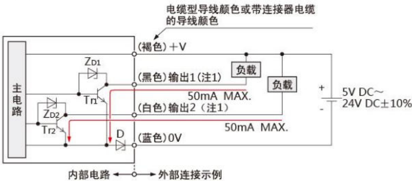
NPN型
