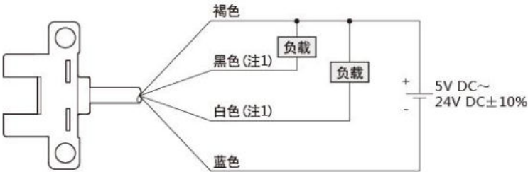
连接图
