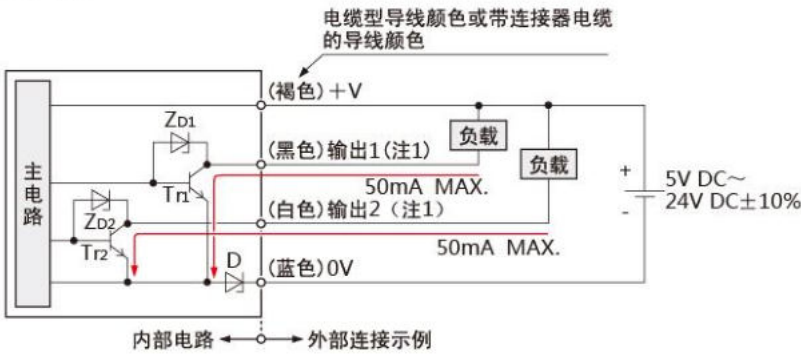
NPN型
